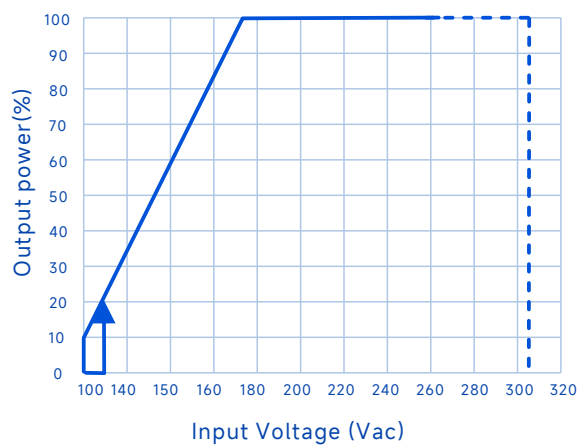
输出功率Vs.输入电压(环温最大55℃)
